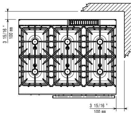
Boven aanzicht
